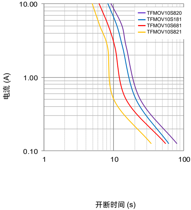
受限电流测试曲线 (UL 1449)
